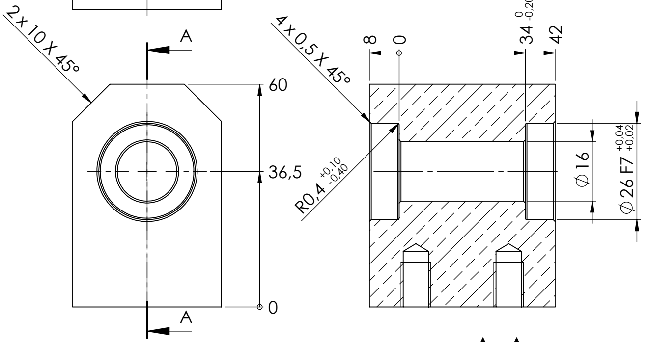
SCHNITT A-A
