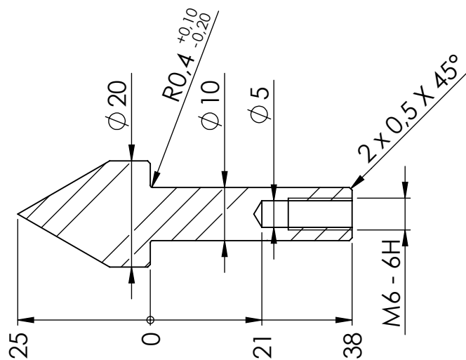
SCHNITT A-A
